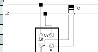
Diagrama Elétrico:
